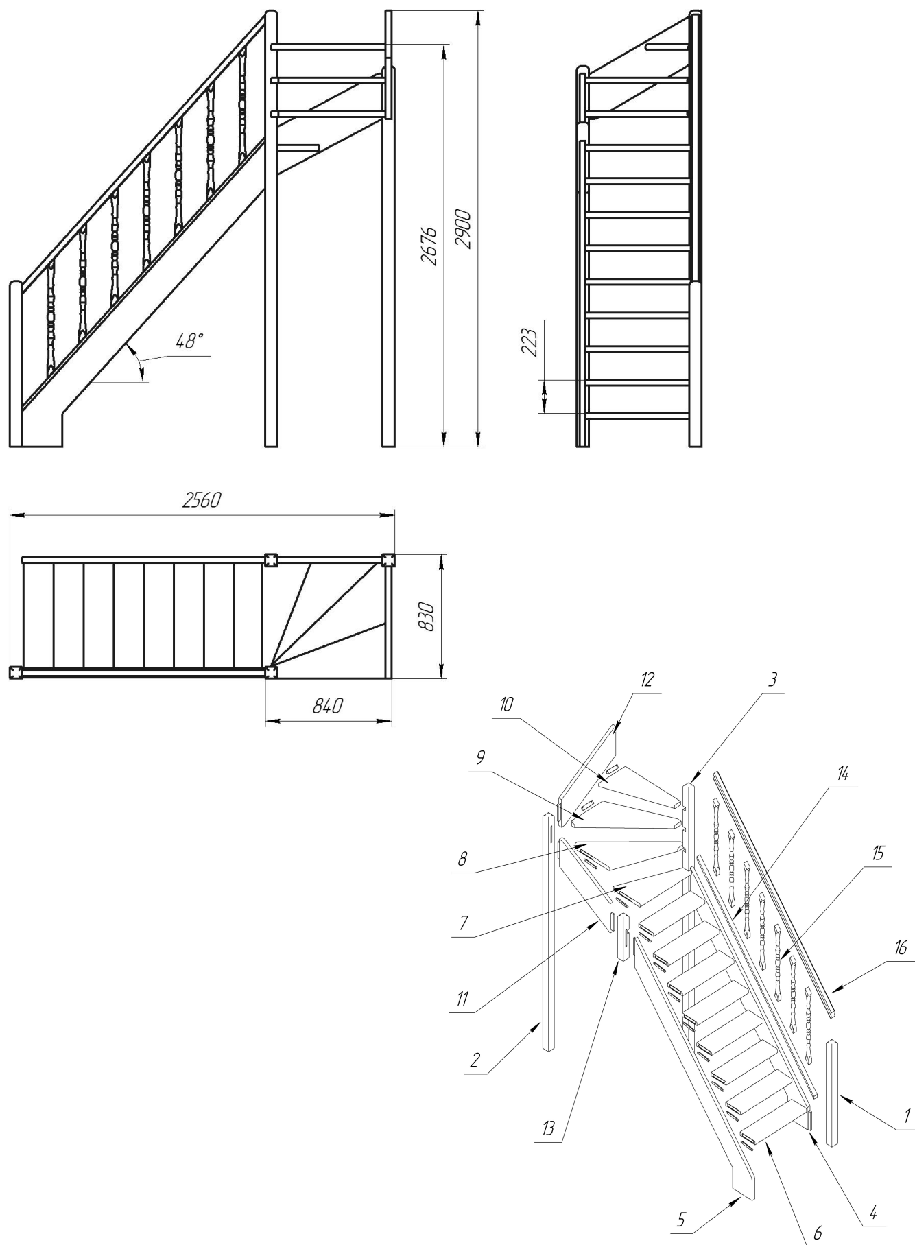
Рисунок 2. Лестница внутриквартирная универсальная ЛЕС-715.
